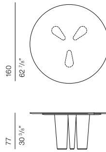
OTT801 table ø160 H77
