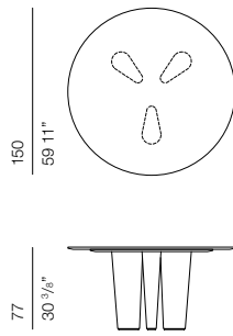
OTT800 table ø150 H77
