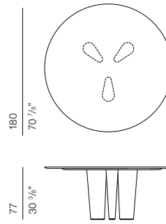
OTT802 table ø180 H77
