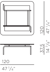
CHA030 low table 120 x 120
