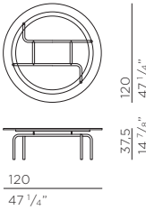
CHA031 low table ø 120
