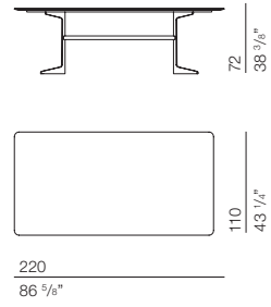
BLA101 table 220 x 110 H72
